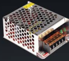
989 25W, IP20 OUTPUT 12V DC 2,1A INPUT ~100-120V 0,6A INPUT ~200-240V 50/60Hz 0,35A
