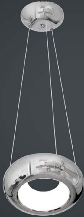
328 12W (85W), 840 Lm, 4000K [REPLACEABLE WYMIENNY] METAL
