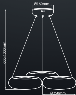
328 12W (85W), 840 Lm, 4000K [REPLACEABLE WYMIENNY] METAL
