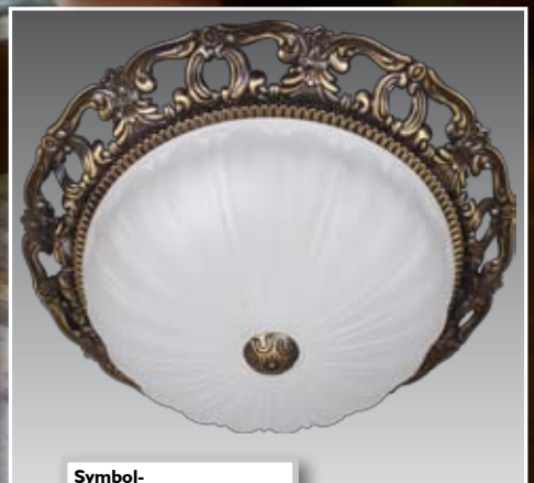
Symbol- ZK-2/766/P 2x E-27, 60W wymiary lampy W=350 H=350 L=110 material-znal. szkło
