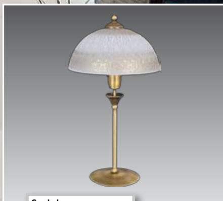
Symbol- S-1/963/P/RUS E-27, 60W wymiary klosza W=300 H=130 wymiary lampy W=300 H=540 material-metal, szkło
